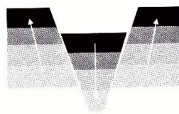
příkopová propadlina
